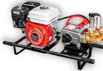
Fumigadoras estacionarias. Motor a Gasolina y Eléctrico.
